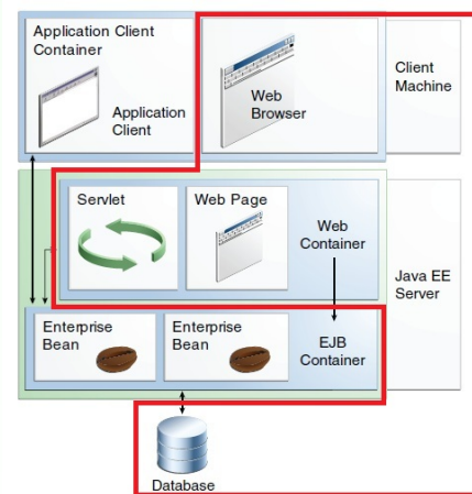
Java EE szerver és konténerek [Java EE Tutorial]
