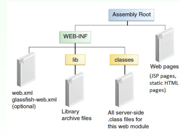
Java EE web modul [Java EE Tutorial]
