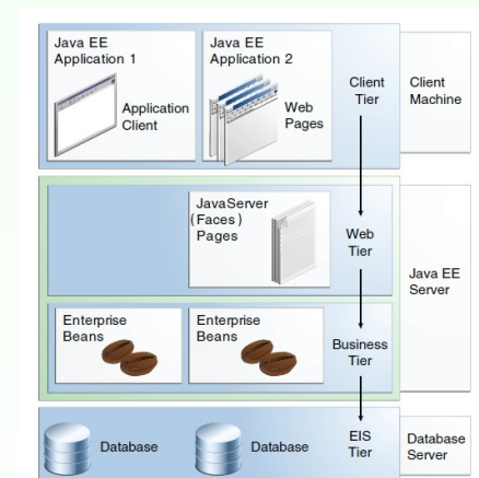
Többrétegű alkalmazások [Java EE Tutorial]
