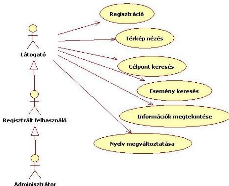
3. ábra: Látogató Use Case Diagram
