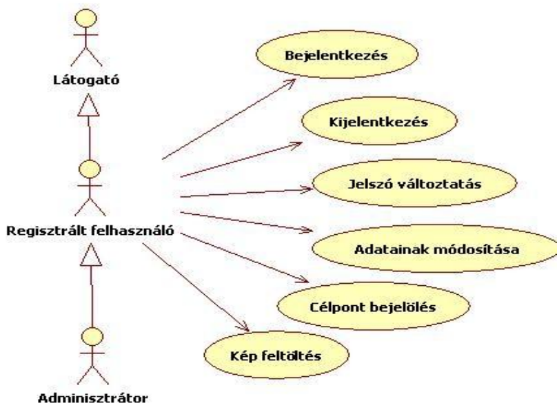
4. ábra: Regisztrált felhasználó Use Case Diagram
