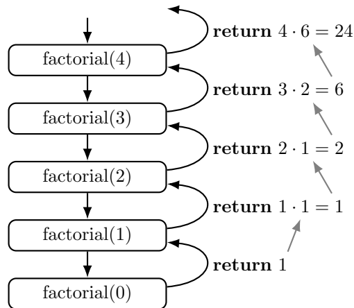
Figura 7.1 Arbore de apeluri recursive pentru calculul lui 4! . Fiecare nod reprezintă un apel al funcției Factorial , care se reduce până când se atinge cazul de bază.
