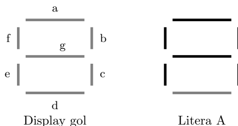
Figura 13.3 Fiecare literă (a,b,c,d,e,f,g) corespunde cu un bit în reprezentarea în baza 2 (de la stânga la dreapta, în ordinea dată). A conține a,b,c,e,f,g , astfel transformarea va genera: 1110111_2 = 119_{10}
